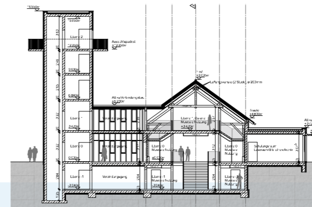
Schnittzeichnung des neuen Kompetenz- und Begegnungszentrum und Späneturm (links).
